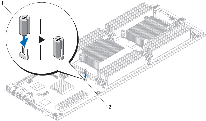
Figure 1. Installation du cavalier en caoutchouc
