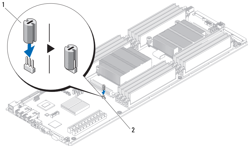
图 1. 安装橡胶跳线
