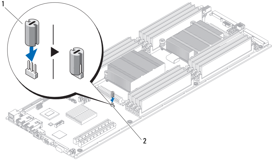
1 고무 점퍼 2 시스템 보드 점퍼 (PCN3)
