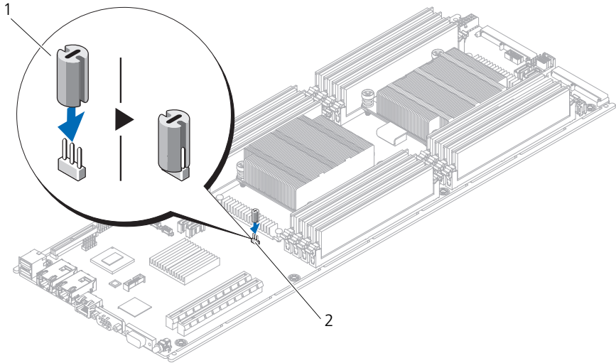
図 1. ゴム製ジャンパの取り付け
